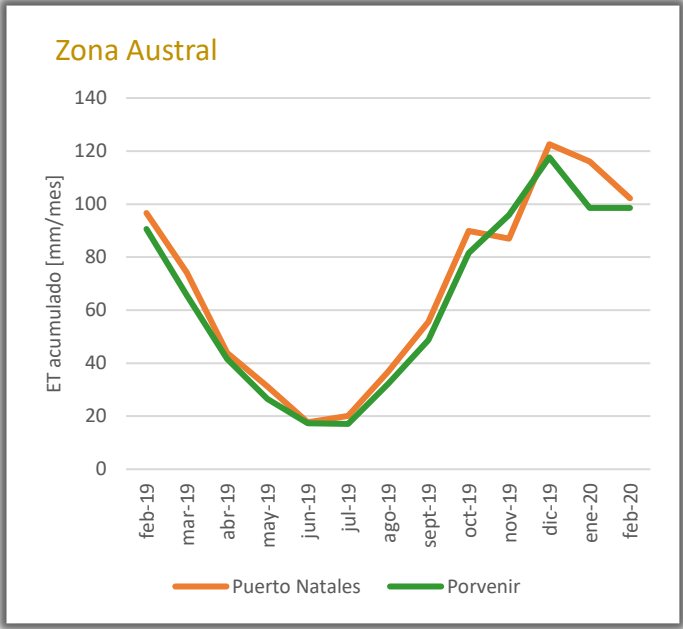
Figura.10 Evapotranspiración acumulada mensual para dos localidades de la Zona Austral. Se muestran los totales mensuales entre febrero de 2019 y febrero de 2020. Datos: DMC.
