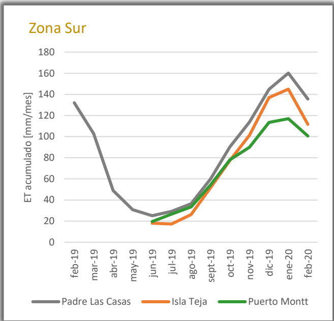
Figura.9 Evapotranspiración acumulada mensual para tres localidades de la Zona Sur. Se muestran los totales mensuales entre febrero de 2019 y febrero de 2020. Datos: DMC.
