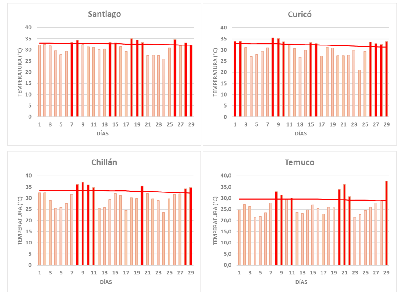
Figura 4b. Evolución diaria de la temperatura máxima de algunas localidades del país durante febrero de 2020. La línea de color rojo indica el percentil 90 (P90) de la temperatura máxima diaria para cada estación. Las barras de color rojo indican los días en que la temperatura máxima superó el percentil 90 Datos: DMC.
