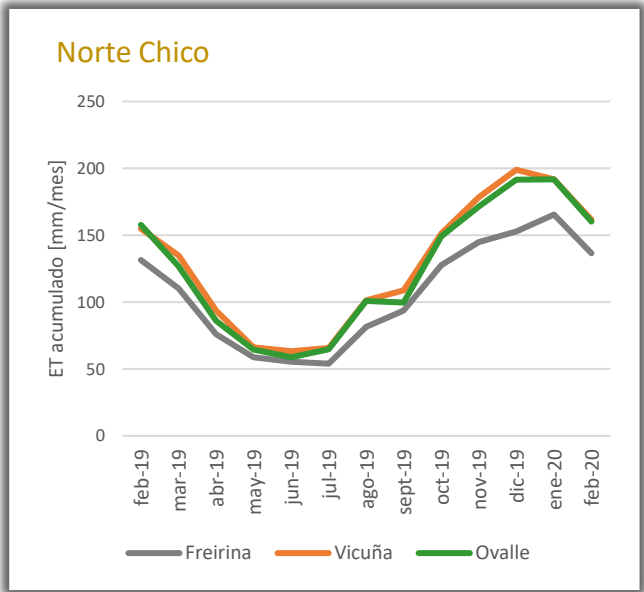
Figura.7 Evapotranspiración acumulada mensual para tres localidades del Norte Chico. Se muestran los totales mensuales entre febrero de 2019 y febrero de 2020. Datos: DMC.
