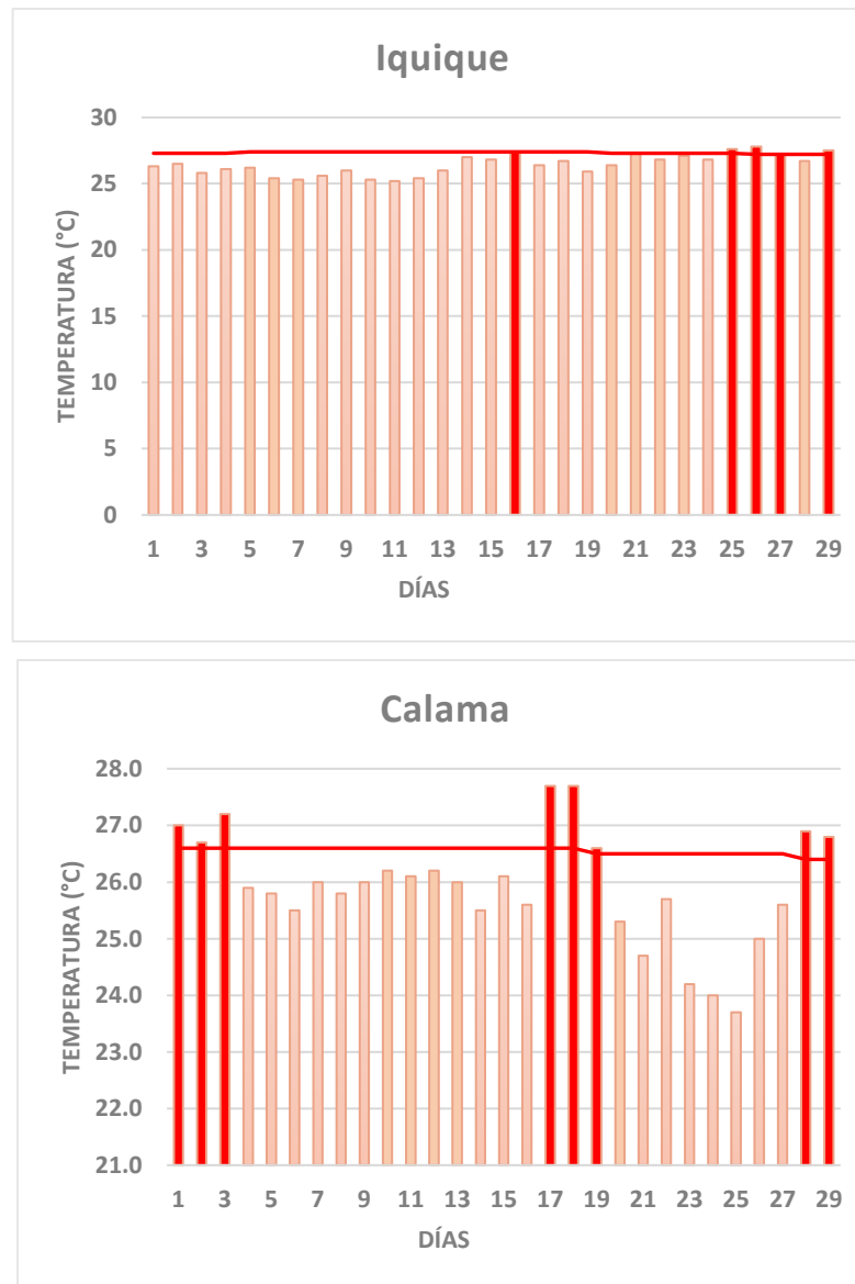
Figura 4a. Evolución diaria de la temperatura máxima de algunas localidades del país durante febrero de 2020. La línea de color rojo indica el percentil 90 (P90) de la temperatura máxima diaria para cada estación. Las barras de color rojo indican los días en que la temperatura máxima superó el percentil 90 Datos: DMC.
