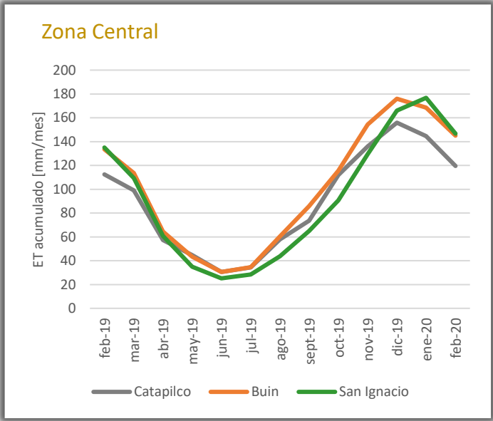
Figura.8 Evapotranspiración acumulada mensual para tres localidades de la Zona Central. Se muestran los totales mensuales entre febrero de 2019 y febrero de 2020. Datos: DMC.
