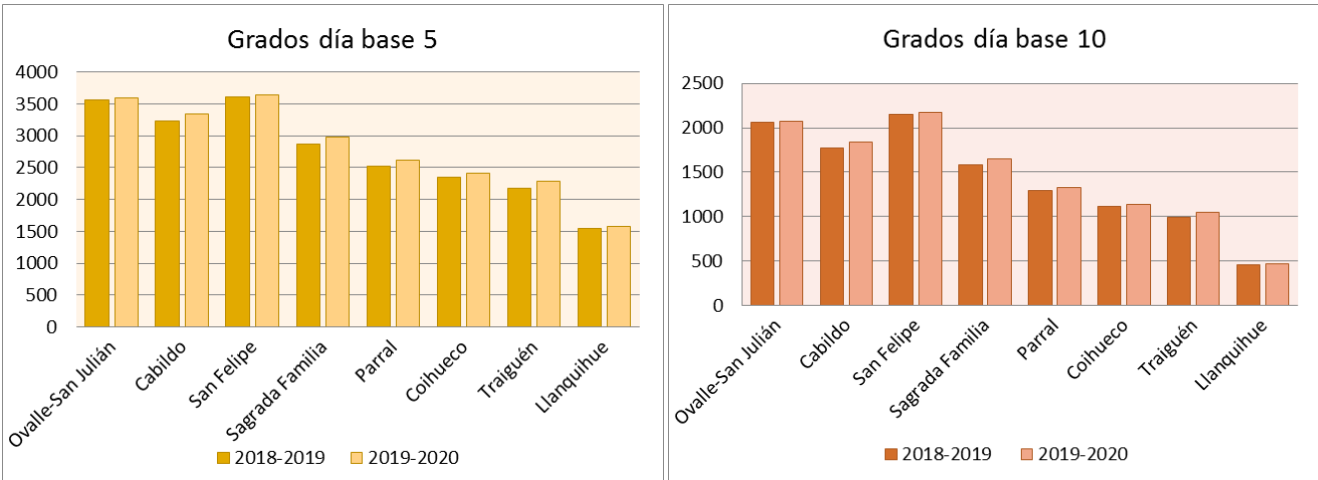
Figura 5. Acumulación de Grados Día (base 5 izquierda y base 10 derecha) para algunas localidades entre las regiones de Coquimbo y Los Lagos, para los períodos 01 de mayo al 29 de febrero de las últimas dos temporadas (2018-2019 / 2019-2020). Datos: RED AGROCLIMA – DMC.
