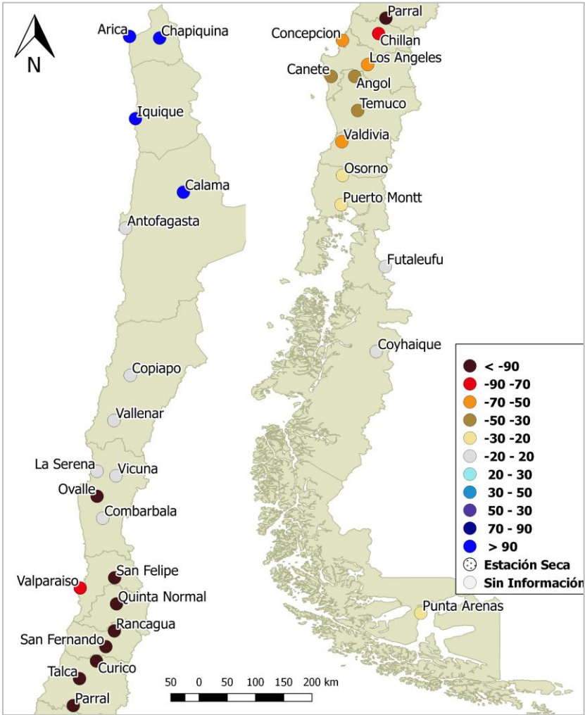
Figura 3. Mapa de déficit y/o superávit (en porcentaje) de precipitación acumulada desde el 01 de enero al 29 de febrero de 2020, para 31 localidades entre las regiones de Arica-Parinacota y Magallanes. La escala de colores, indicadas por círculos, representa el porcentaje de déficit o superávit de lluvia acumulada con respecto a un año normal. Período climático base: 1981-2010. Datos: DMC-DGA-SERVIMET.
