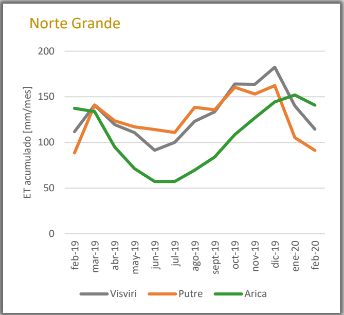
Figura.6 Evapotranspiración acumulada mensual para tres localidades del Norte Grande. Se muestran los totales mensuales entre febrero de 2019 y febrero de 2020. Datos: DMC.
