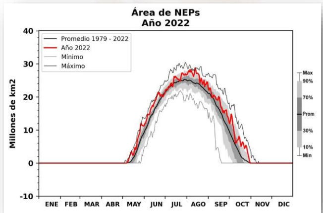
Figura 14. Área de Nubes Estratosféricas Polares Tipo I. Fuente: NASA
