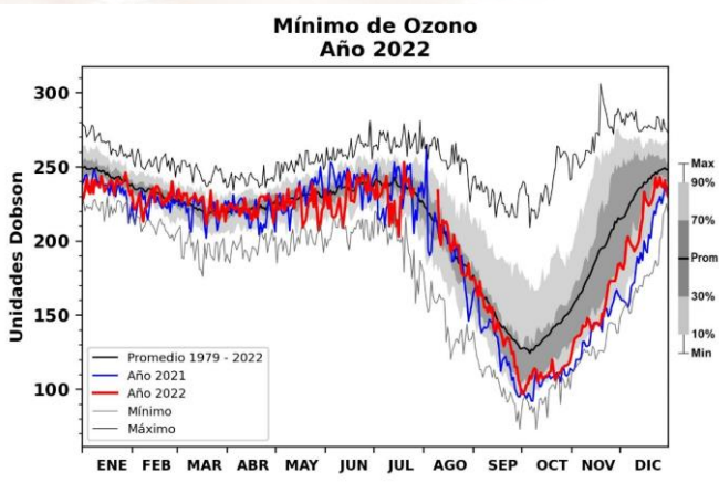
Figura 2. Mínimo de columna de ozono en unidades Dobson (DU). Fuente: NASA.
