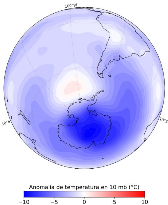
Figura 8. Anomalía de temperatura en los 10 mb durante septiembre, octubre y noviembre de 2022. Período de referencia para el cálculo de anomalía 1991-2020. Fuente: Reanálisis NCEP/NCAR.
