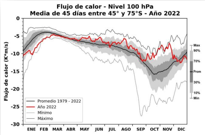
Figura 12. Flujo longitudinal de calor en el nivel de 100 hPa, expresado en K*m/s. Mientras mas negativos los valores, mayor flujo de calor. Fuente: NASA
