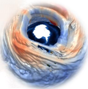
Figura 3. Agujero de Ozono el día 15 de octubre de 2022. Fuente: Programa Copernicus.
