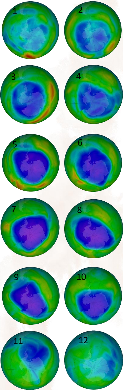
Figura 17. Columna de ozono total para los días 1) 01-agosto, 2) 15-agosto, 3) 30-agosto, 4) 01-septiembre, 5) 15-septiembre, 6) 01-octubre, 7) 15-octubre, 8) 31-octubre, 9) 02-noviembre, 10) 15-noviembre, 11) 30-noviembre y 12) 15-diciembre de 2022. Fuente: NASA.
