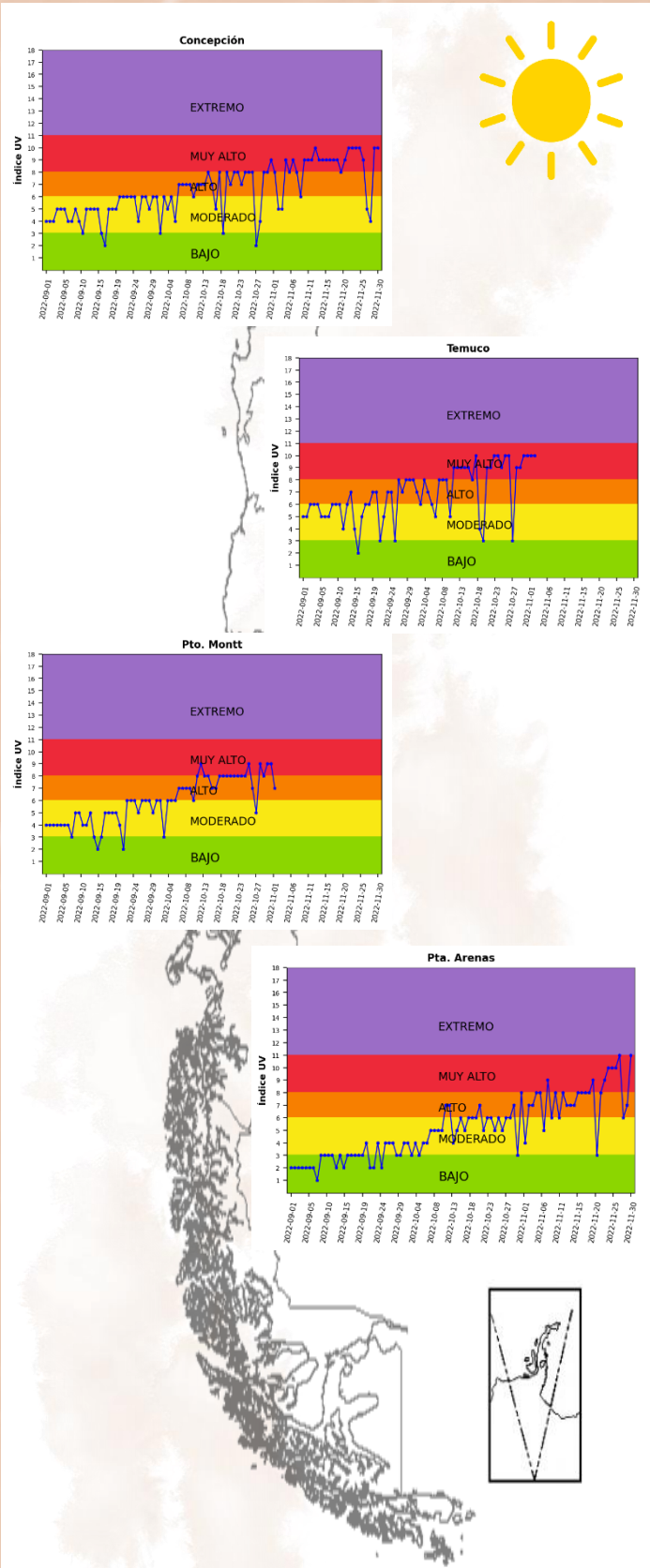
Figura 16. Valores de Índice Ultravioleta durante septiembre a noviembre de 2022 en ciudades del sur del país. Fuente: DMC
