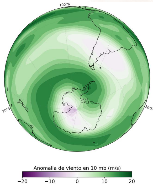
Figura 9. Anomalía de viento zonal en los 10 mb durante septiembre, octubre y noviembre de 2022. Período de referencia para el cálculo de anomalía 1991-2020. Fuente: Reanálisis NCEP/NCAR.
