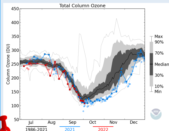
Figura 1. Columna de ozono total (en [UD]) en promedio para el Polo Sur. Los datos están desde el mes de julio y es posible comparar con año anterior (2021). Fuente: NOAA.
