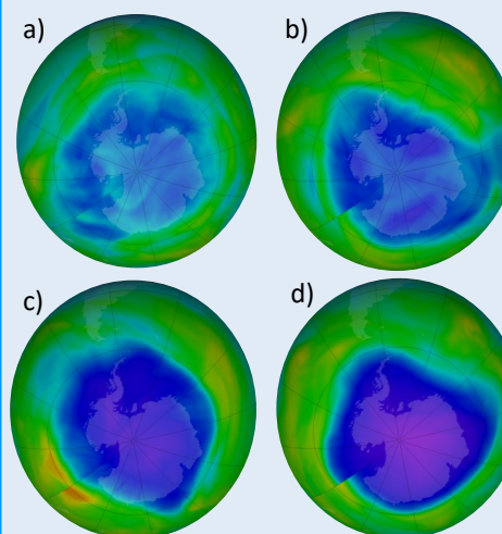
Figura 2. Columna de ozono total para los días a) 15-agosto, b) 01-septiembre, c) 15-septiembre y d) 30-septiembre de 2022. Fuente: NASA.
