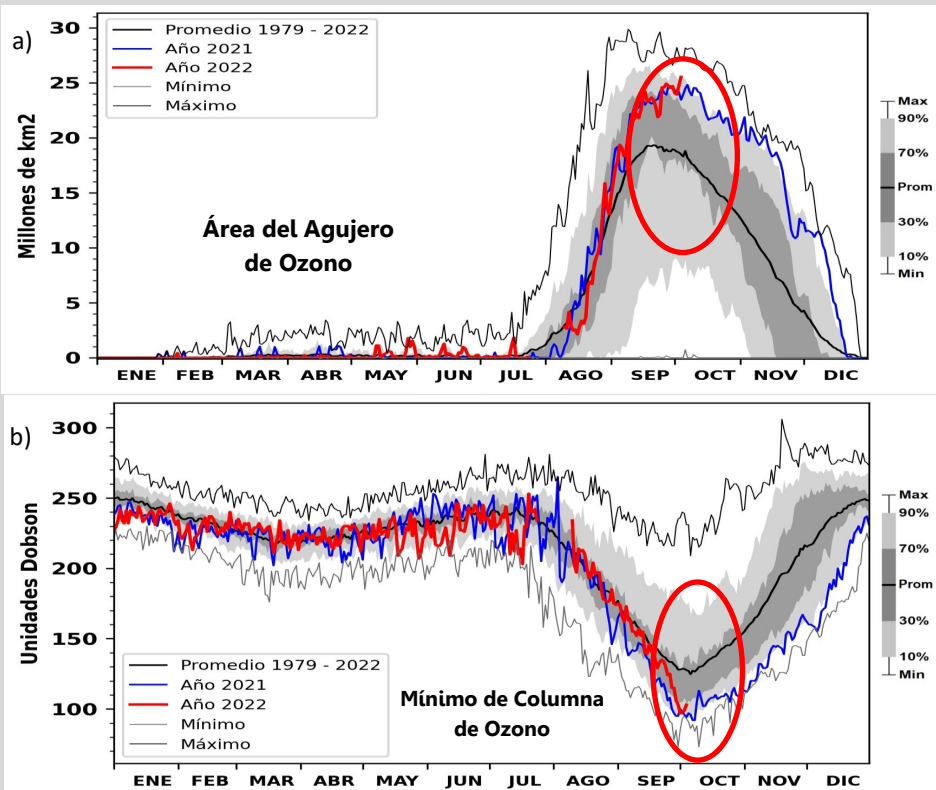
Figura 4. a) Área y b) Mínimo de columna de Ozono en Unidades Dobson [UD] para latitudes mayores de 30°S. Fuente: NASA Ozone Watch.
