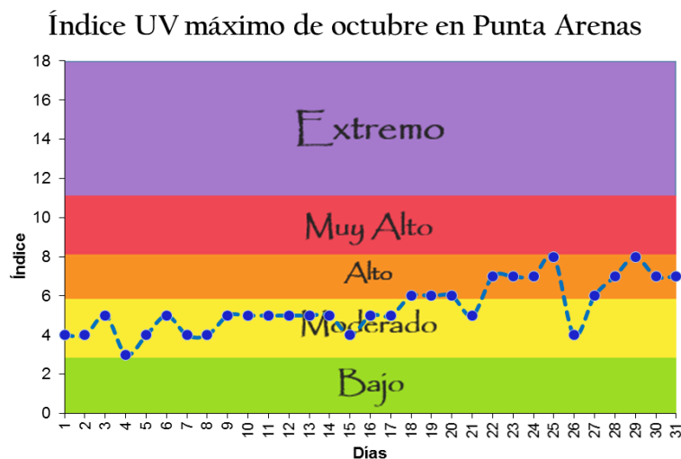
Figura 9.— Índice de Radiación Ultravioleta máximo del día en la estación Antártica Eduardo Frei.
